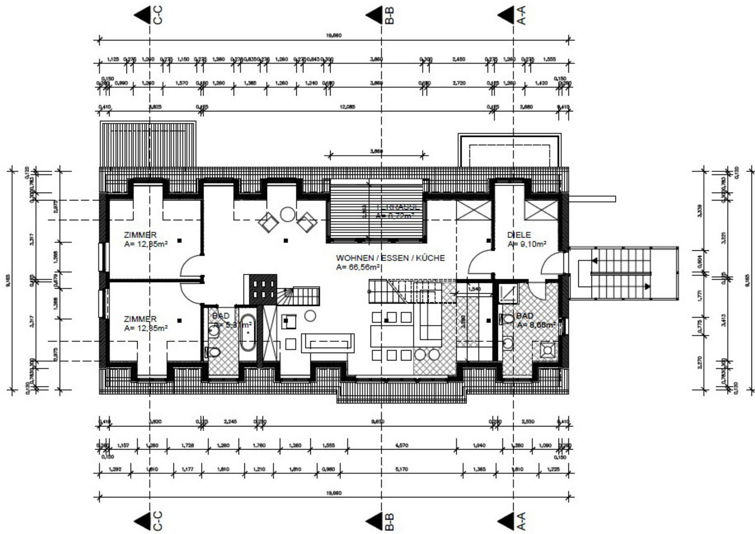
GRUNDRISS DG
